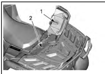
1. Защелка перчаточного ящика 2. Отверстия системы «LINQ»
