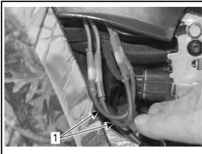
1. Перемычки
