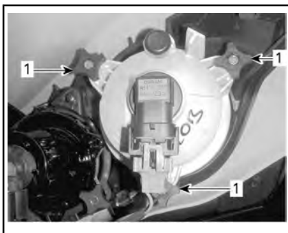
РЕГУЛИРОВКА БЛИЖНЕГО СВЕТА ФАР
