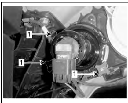
РЕГУЛИРОВКА ДАЛЬНОГО СВЕТА ФАР
