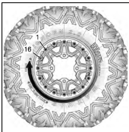
ТИПОВОЙ ВАРИАНТ - ЗАКЛЮЧИТЕЛЬНЫЙ ЭТАП ЗАТЯЖКИ ВИНТОВ
