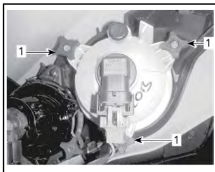
ロービーム調整
