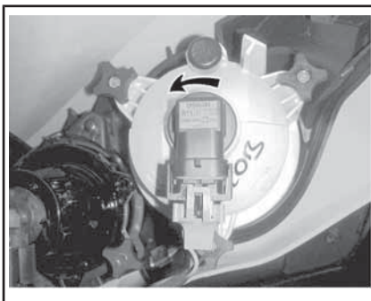
DIMLICHTEN
