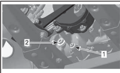
TYPISCH - 650 MOTOR
