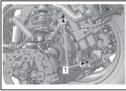
WIELDRAAGARMEN VOORAAN
