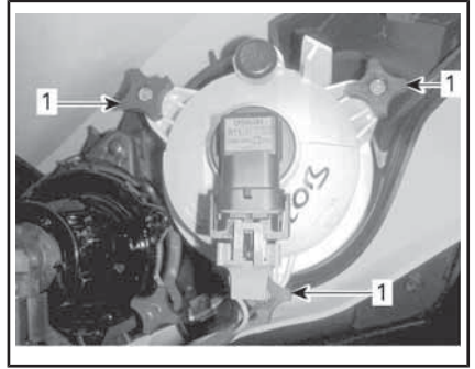
DIMLICHT REGELEN
