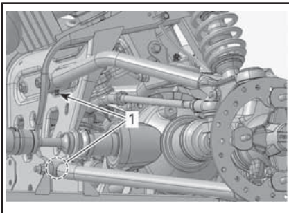
OPHANGINGSARMEN ACHTER
