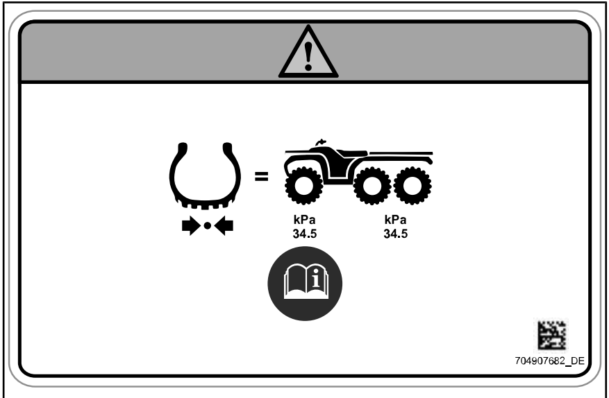
HINWEISSCHILD 4
