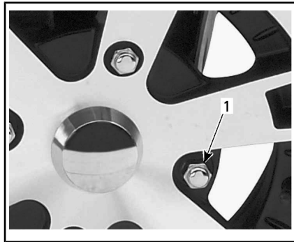
TYPISCH — ALUMINIUMRAD
