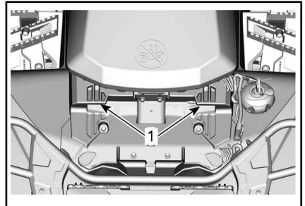
1. Vordere Raststifte
