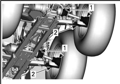
TYPISCH — FAHRZEUGRÜCKSEITE
