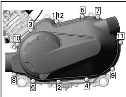
CVT-ABDECKUNG-ANZUGSREIHENFOLGE
