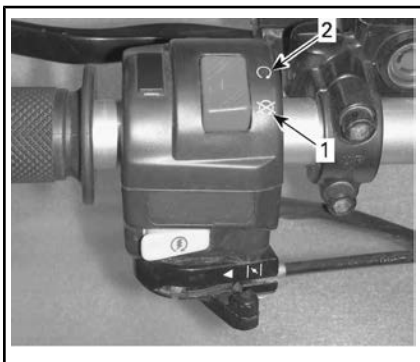
TÍPICA - INTERRUPTOR DE PARADA DE EMERGÊNCIA DO MOTOR
