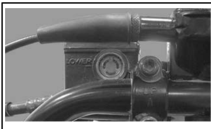
RESERVATÓRIO DIREITO, DO FLUIDO DO FREIO DIANTEIRO
