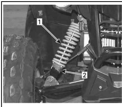
DS 70 E DS 90 — SUSPENSÃO DIANTEIRA
