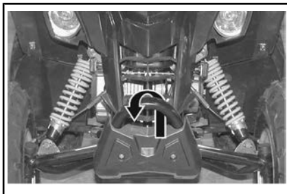
DS 70 E DS 90 — PONTOS DE FIXAÇÃO NA DIANTEIRA
