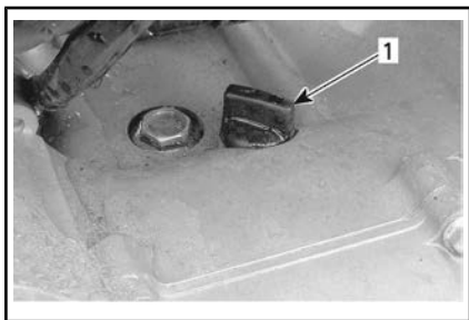
BUJÃO DE ENCHIMENTO — LADO ESQUERDO DO MOTOR
