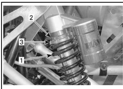
DS 90 X — SUSPENSÃO DIANTEIRA
