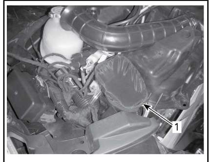
1. CVT-luchtfilter
