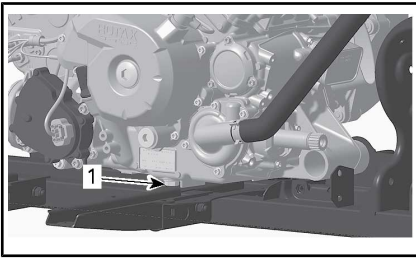
1. Afvoerplug
