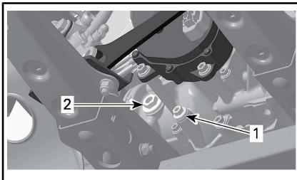
CONFIGURAZIONE TIPICA - MOTORE 570/850
