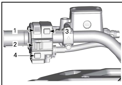
CONFIGURAZIONE TIPICA — INTERRUITTORE MULTIFUNZIONE
