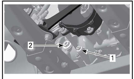
CONFIGURAZIONE TIPICA - MOTORE 570/650/850
