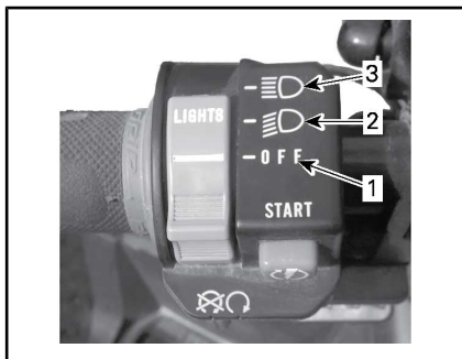
FUNZIONI DELL'INTERRUPTORE DEL FARO
