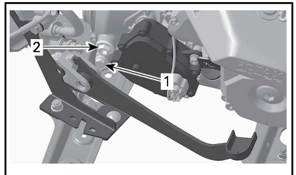
CONFIGURAZIONE TIPICA - MOTORE 1.000R
