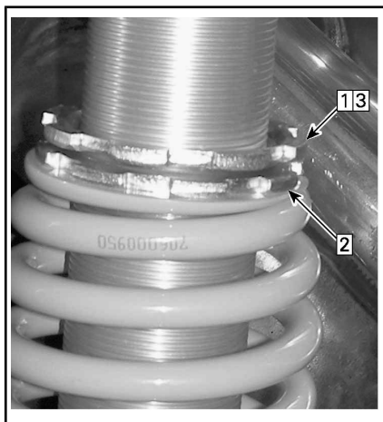
TÍPICO 850 E 1000R
