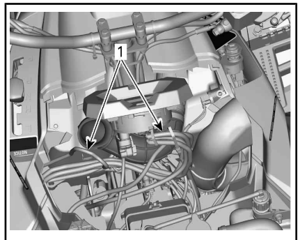
TÍPICO - SUPORTE DO INDICADOR REMOVIDO PARA MELHOR VISUALIZAÇÃO - MODELOS 570, 650 E 850
