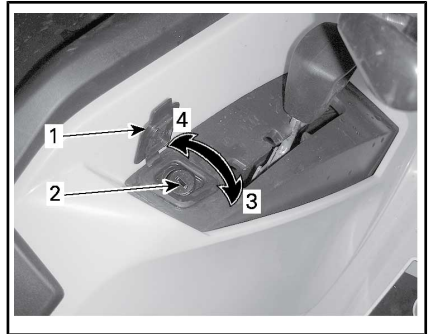
VERGRENDELMECHANISME SCHAKELHENDEL
