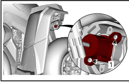
TYPISCH - LAMPJE RICHTINGAANWIJZER VOORAAN
