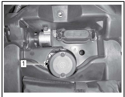
1. Achterrem-vloeistofreservoir
