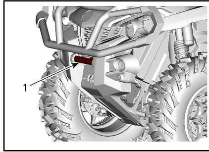
1. Vorderer Verzurppunkt
