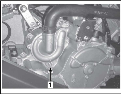
1. Jäähdytysnesteen tyhjennystulppa
