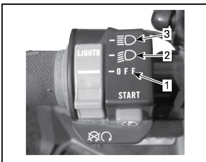
FUNCTIES VAN DE DIMSCHAKELAAR
