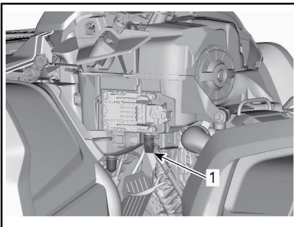
1. Toevoerbuus van het luchtfilterhuis
