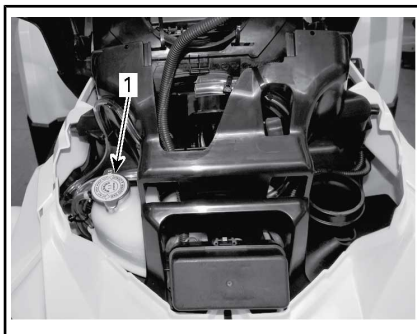
1. Dop motorkoelvloeistoftank
