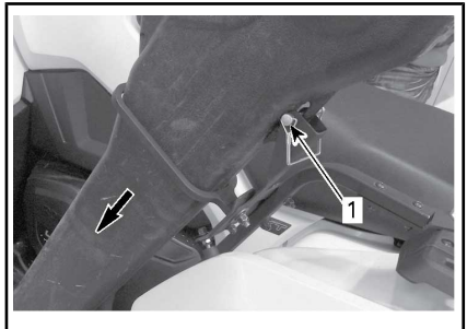
1. Perno bloccato
