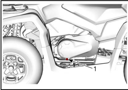
1. CVT-aftapplug
