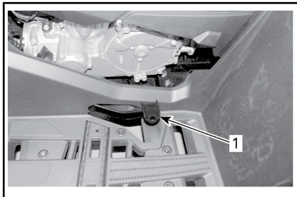
1. Rempedaal
