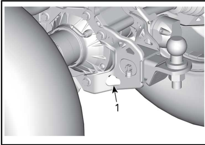
TYPISCH - BEVESTIGINGSPUNT ACHTERAAN
