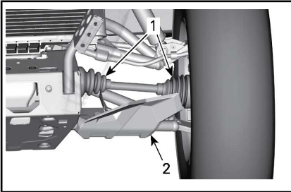
TYPISCH — FAHRZEUGVORDERSEITE
