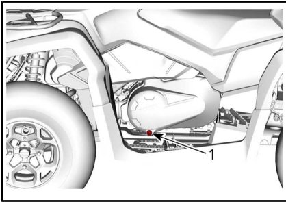
1. CVT-Ablassstopfen
