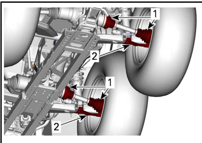
TYPISCH — FAHRZEUGRÜCKSEITE
