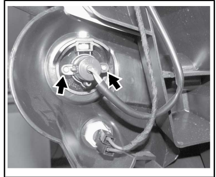
DESATORNILLE LOS TORNILLOS DE FIJACIÓN DE LA BOMBILLA DEL INTERMITENTE DELANTERO
