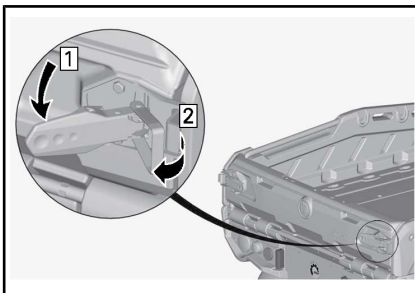
2. Baje la puerta trasera
