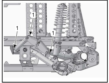
BARRA ESTABILIZADORA
