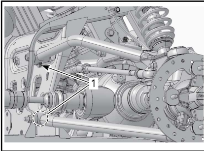
BRAZOS DE LA SUSPENSIÓN TRASERA
