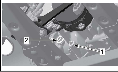
TÍPICO - MOTOR 650
