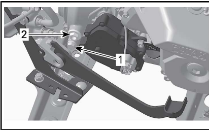
TÍPICO - MOTOR 1000
