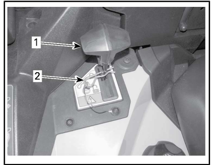
1. Mango (tirador) de desbloqueo 2. Pasador de horquilla
