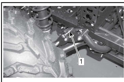
1. Pasador de la barra estabilizadora bloqueado
