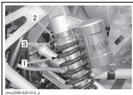
DS90 X — ПЕРЕДНЯЯ ПОДВЕСКА
