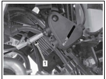
EINSTELLUNG VOM GASZUGBEGRENZUNGSFACH ZUM MOTOR
