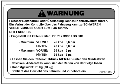
HINWEISSCHILD 4 - TYPISCH
