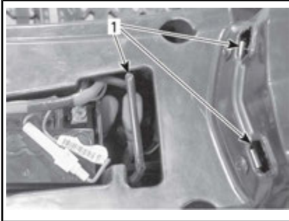
1. Haken
