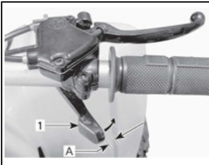
TYPISCH — NORMALES SPIEL
