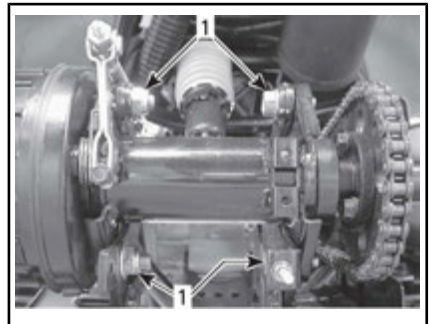
TYPISCH — HINTERACHSE
