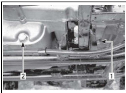
ABLASSSCHRAUBE — LINKE MOTORSEITE
