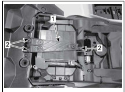
1. Accuhouder 2. Borgschroeven
