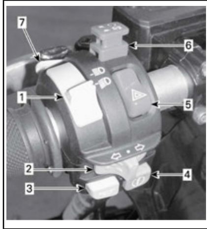
TÍPICO - INTERRUPTOR MULTIFUNCIÓN
