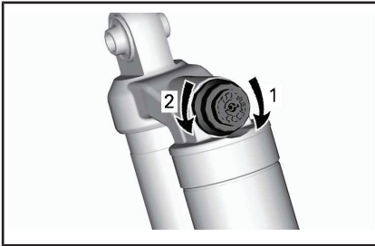
AMORTIGUACIÓN DE COMPRESIÓN - PARTE SUPERIOR DEL AMORTIGUADOR
