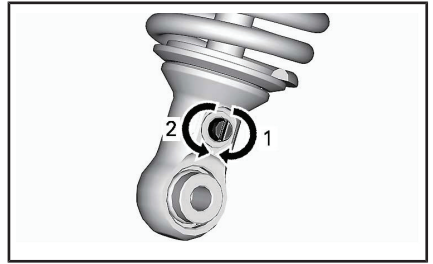
AMORTIGUACIÓN DE REBOTE - PARTE INFERIOR DEL AMORTIGUADOR
