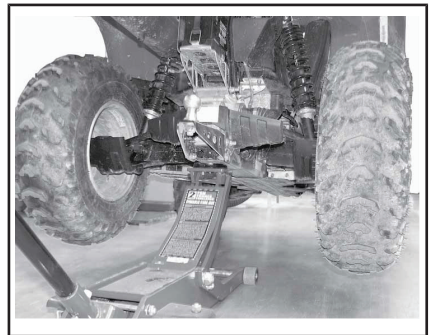
TYPEBILDE – LØFTEPUNKT BAK PÅ KJØRETØYET
