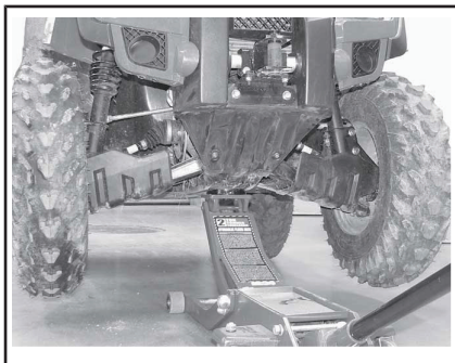
TYPIQUE — POINT DE LEVAGE AVANT
