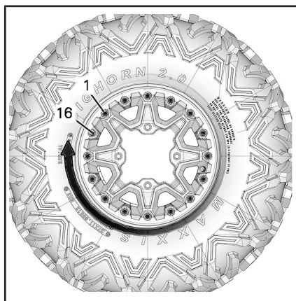
TYPIQUE - SÉQUENCE DE SERRAGE FINAL
