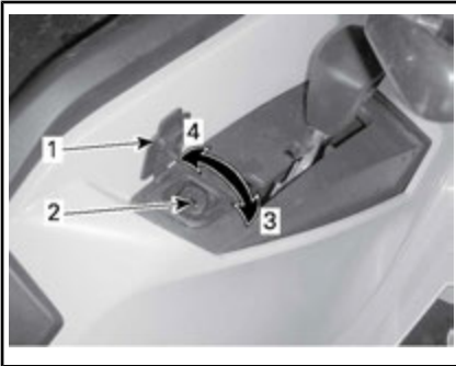
SCHALTHEBEL-VERRIEGLUNGSMECHANISMUS
