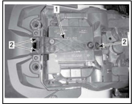
1. Batteriebügel 2. Halteschrauben
