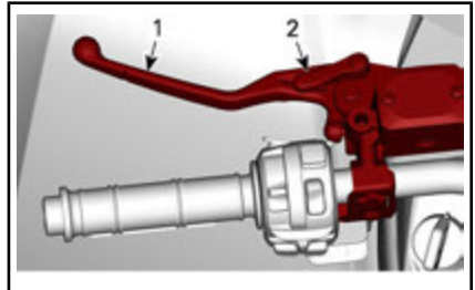
1. Bremshebel 2. Arretierung
