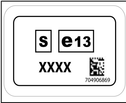
AUF ANHÄNGERKUPPLUNG
