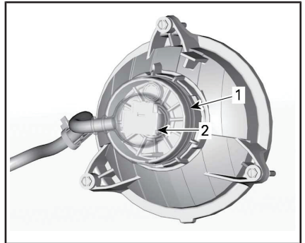
1. Achterste zekerbare aansluitingen en zekeringhouder(s)
