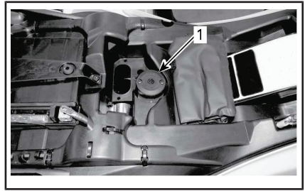
1. Achterrem-vloeistofreservoir
