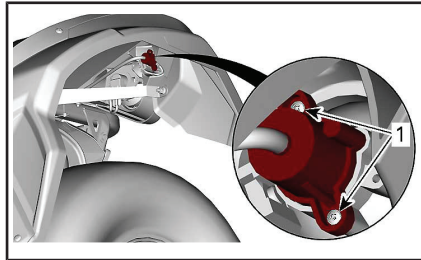
TYPISCH - LAMPJE RICHTINGAANWIJZER ACHTERAAN
