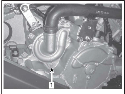
1. Koelvloeistofaftapplug
