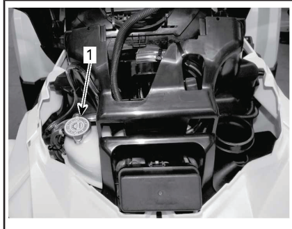
1. Moottorin jäähdytysnestesäiliö
