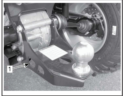
TYYPILLINEN – KIIINNITYSKOHTA TAKANA
