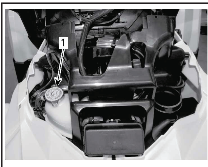
1. Motorkühlmittelbehälter
