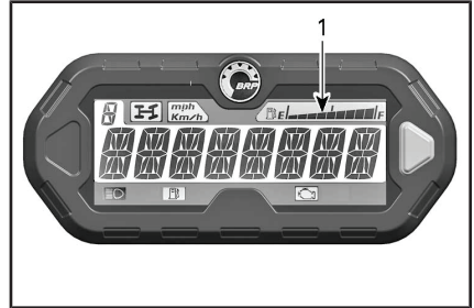
1. Kraftstoffstandanzeige
