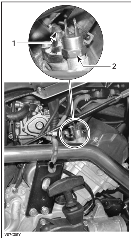
V07C09Y 1. Vis de purge 2. Sonde de température du moteur
