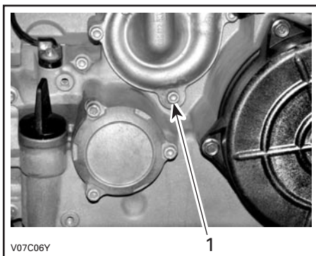
V07C06Y 1. Bouchon de vidange de liquide de refroidissement
