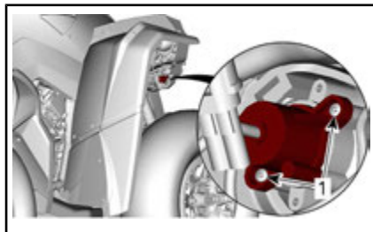
TYPISCH - LAMPJE RICHTINGAANWIJZER VOORAAN
