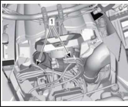
TÍPICO - PIEZAS DEL SOPORTE DEL INDICADOR RETIRADAS PARA MAYOR CLARIDAD - MODELOS 570, 650 Y 850
