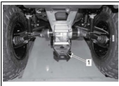
1. Bärningskrok
