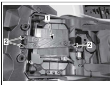
1. Batterihållare 2. Hållskruvar
