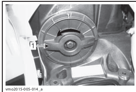
1. Крышка корпуса воздушного фильтра
