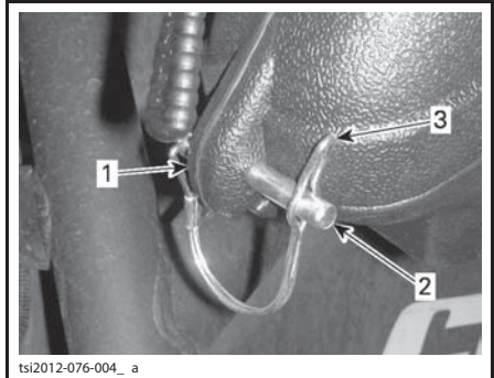
1. Задняя часть оружейного кофра 2. Палец 3. Фиксатор
