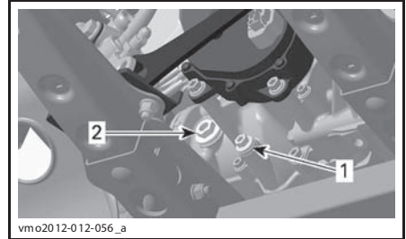
1. Пробка сливного отверстия 2. Пробка для проверки уровня масла
