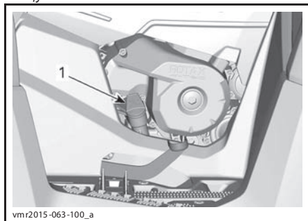
МОДЕЛИ 570 – ПРАВАЯ СТОРОНА ДВИГАТЕЛЯ 1. Щуп
