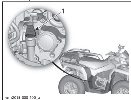
МОДЕЛИ 450 – ПРАВАЯ СТОРОНА ДВИГАТЕЛЯ 1. Щуп
