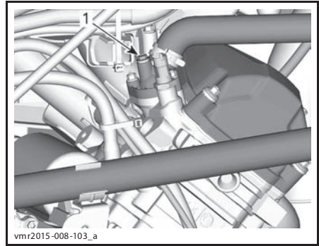
ТИПОВОЙ ВАРИАНТ 1. Сливной винт переднего цилиндра
