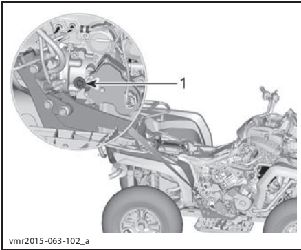
1. Пробка для проверки уровня масла
