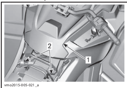
МОДЕЛИ 570 – ПРАВАЯ СТОРОНА ДВИГАТЕЛЯ 1. Щуп
