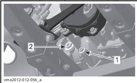
1. Сливная пробка 2. Пробка отверстия для проверки уровня масла
