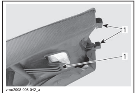
1. Крюки сиденья
