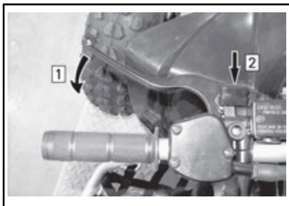
ALAVANCA ESQUERDA DO FREIO
