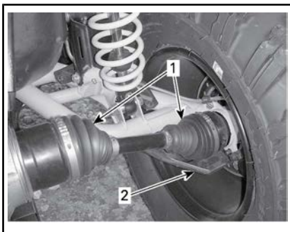
TYPISCH — FAHRZEUGRÜCKSEITE
