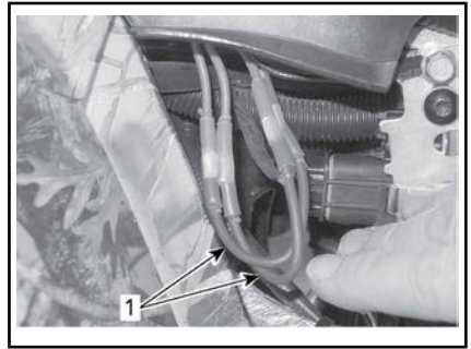
1. Sicherungseinsätze
