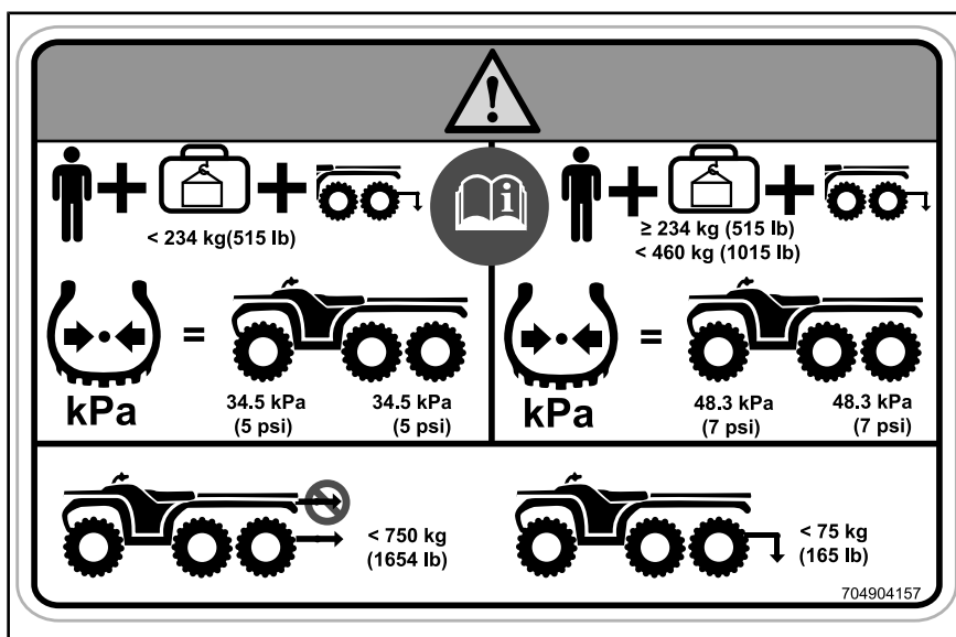
HINWEISSCHILD 8
