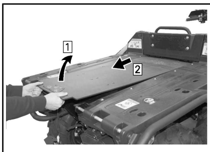
VORDERER GEPÄCKTRÄGER
