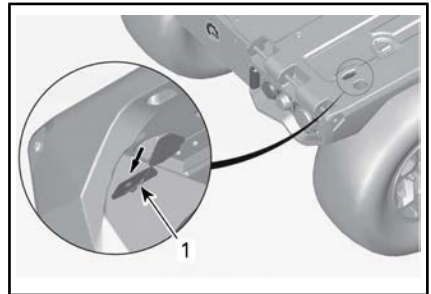
1. Befestigungsplatte
