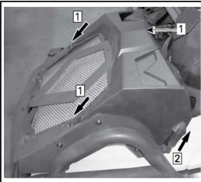
Stap 1: Schuif de lipjes van de radiatorkap Stap 2: Vergrendel de zijanten 1. Radiatorkap
