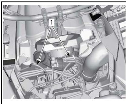
TYPISCH - CONSOLESTEUN VERWIJDERD VOOR DE GOEDE ZICHTBAARHEID - 570-, 650- EN 850-MODELLEN
