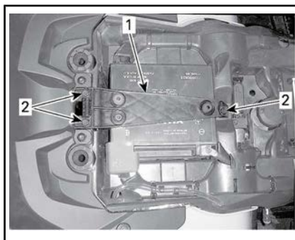
1. Accuhouder 2. Borgschroeven
