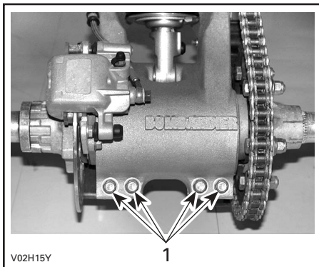
1. Bakaxelns låsbultar
