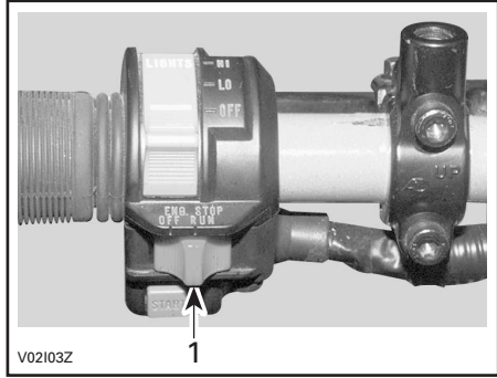
1. Motorns stoppreglage
