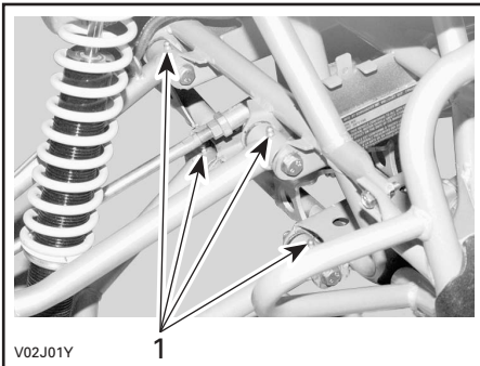
1. Smörjnipplar
