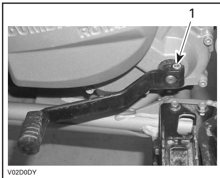
1. Hylsskruv
