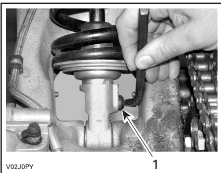
1. Justeringsskruv
