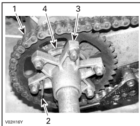
1. Chaîne d'entraînement 2. Loquet de tendeur 3. Moyeu de pignon 4. Carter d'essieu excentrique
