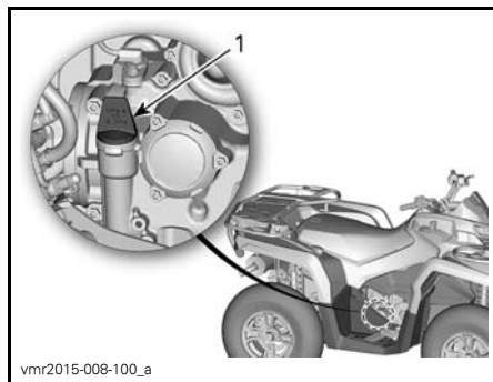
450-MODELL – HØYRE SIDE AV MOTOREN 1. Peilestav
