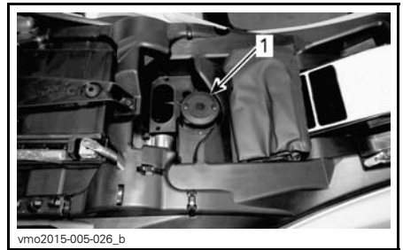
1. Bremsevæskebeholder for bremses bak
