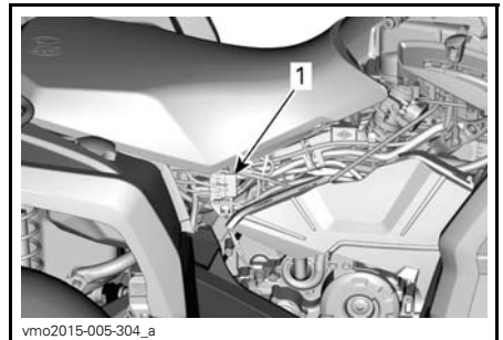
1. Sikringsholder bak
