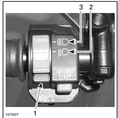
FONCTIONS DU COMMUTATEUR DE PHARE
