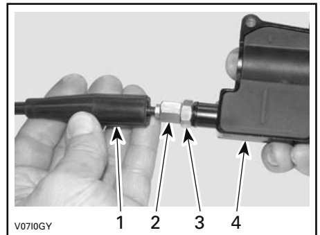
1. Protecteur de câble 2. Dispositif de réglage de câble d'accélérateur 3. Écrou de blocage 4. Logement de manette d'accélérateur
