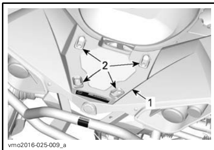
1. Zone de chargement 2. Oeillets en plastique
