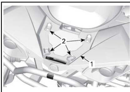
1. Área de carga 2. Ojales de plástico
