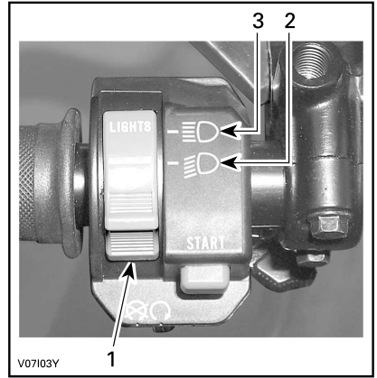
FUNCIONES DEL INTERRUPTOR DE LOS FAROS
