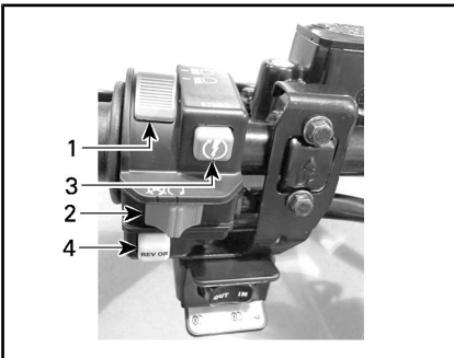
TÍPICO—INTERRUPTOR MULTIFUNCIÓN
