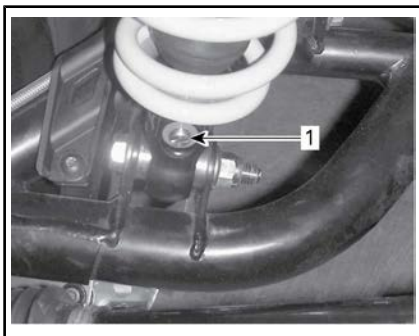
1. Ajustador del rebote (con destornillador plano)
