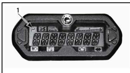
1. Posición de la transmisión
