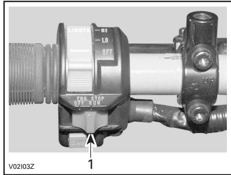
1. Interruptor de paro del motor
