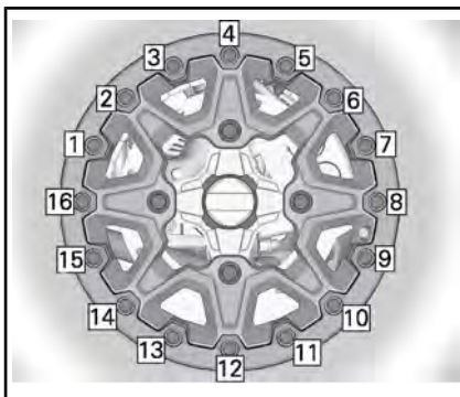
TÍPICO - SEQUÊNCIA FINAL DE APERTO
