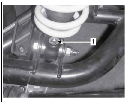
1. Ajustador do rebote (necessário usar chave de fenda)
