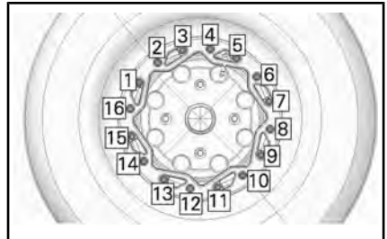
TÍPICO - SEQUÊNCIA FINAL DE APERTO
