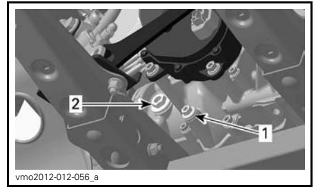
TYPIQUE - MOTEUR 570/850
