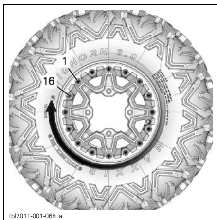
ORDRE DE SERRAGE FINAL TYPIQUE
