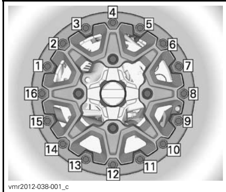
TYPIQUE - ORDRE DE SERRAGE FINAL
