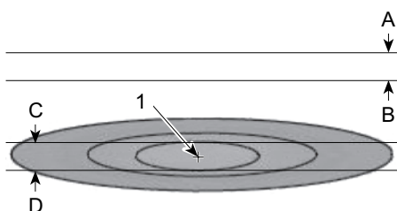
TYPISCH – LICHTBUNDEL VAN DE GROOTLICHTEN OP HET TESTOPPERVLAK – DIMLICHT
