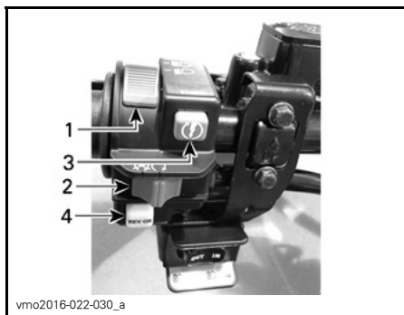
TYPBILD — FLERFUNKTIONSREGLAGE
