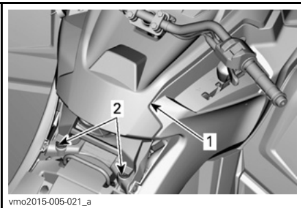
450-MODELL – HÖGER SIDA AV MOTORN 1. Oljemätsticka
