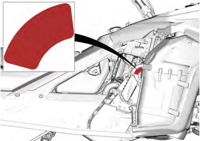
DEKALPLACERING
