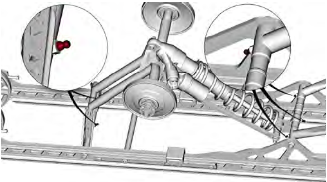
TMOTION XT
