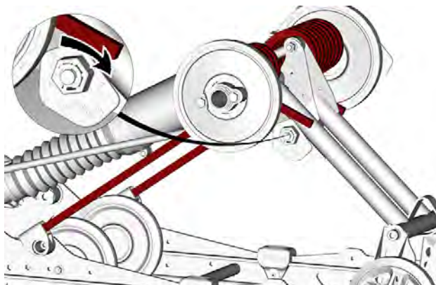
EINSTELLUNG FEDERVORSPANNUNG LINKS – TYPISCH
