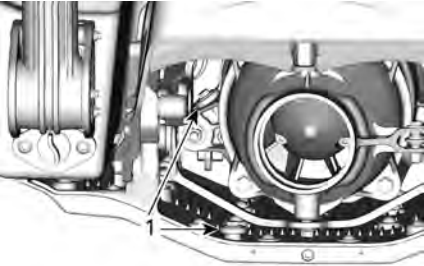
1. 牺牲阳极
